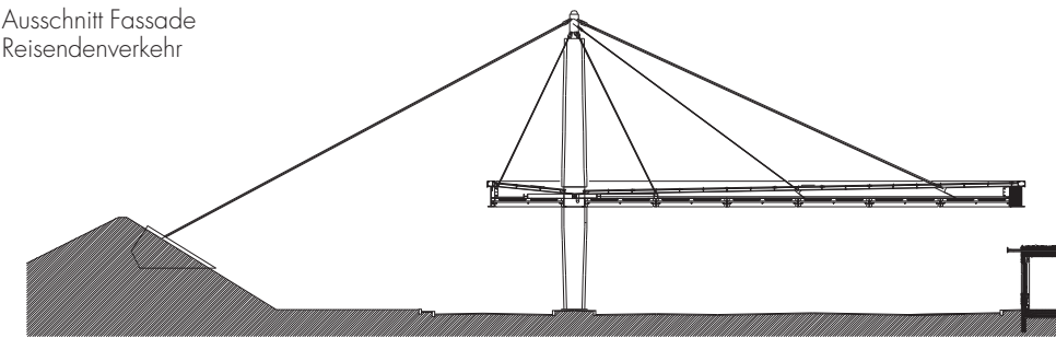
Querschnitt Fahrbahnüberdachung
