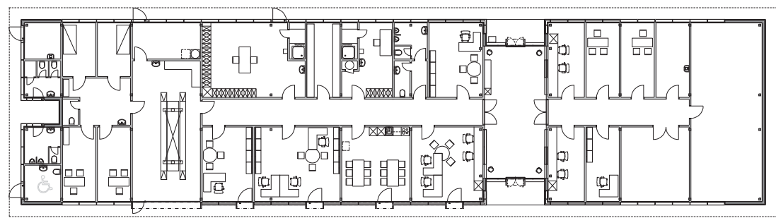
Grundriss / Westfassade Reisendenverkehr
