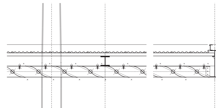
Detail Licht-Umlenk-Lamellen aus rund gewalztem Edelstahlblech
